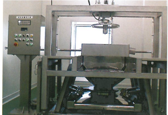
投入ホッパー
