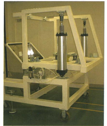
移動式ティルト装置
