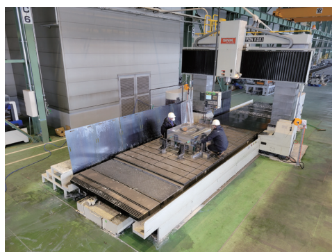
五面加工機
